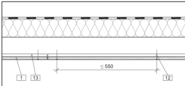
Querschnitt B-B
