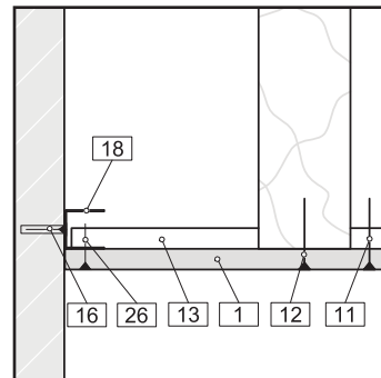
Wandanschluss, Var. 2
