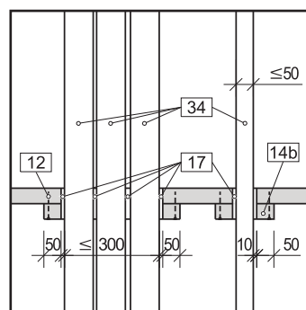
[11] Kabelausgänge Schnitt
