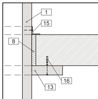
[15] Deckendurchführung, Var. 2
