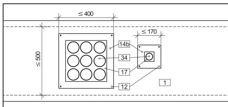
[10] Kabelausgänge Ansicht
