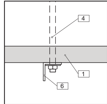
[7] Abhängung, Var. 1
