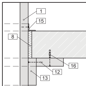
[13] Deckendurchführung
