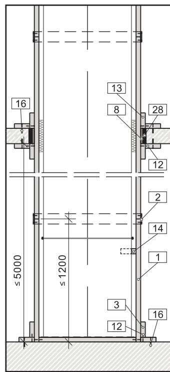
[15] Vertikale Lüftungsleitung, Deckendurchführung / Bodenanschluss
