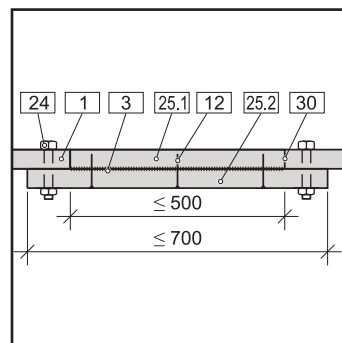
[21] Aufbau Zugangsplatte
