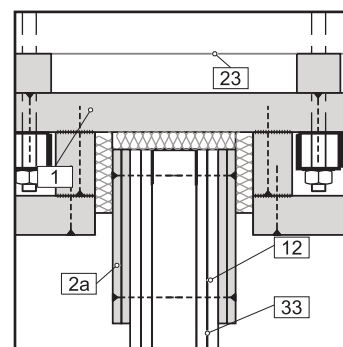
[19] Wanddurchführung Variante
