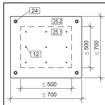
[19] Ansicht Zugangsplatte
