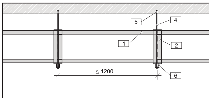
[6] Längsschnitt
