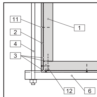
[4] Detail A: Eckausbildung unten
