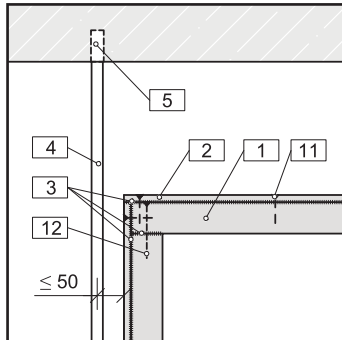
[5] Eckausbildung oben
