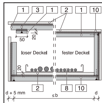
[3] Details: Varianten mit Deckel
