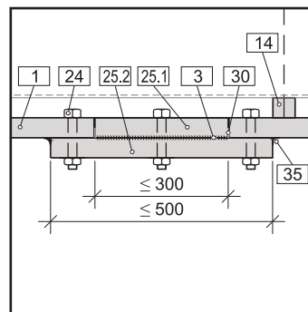
[12] Aufbau Revisionsöffnung
