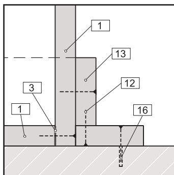
[14] Detail: Bodenanschluss
