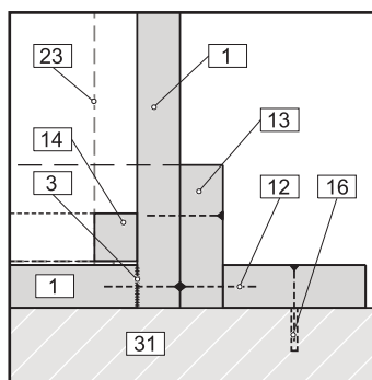
[19] Bodenanschluss, Var. 1
