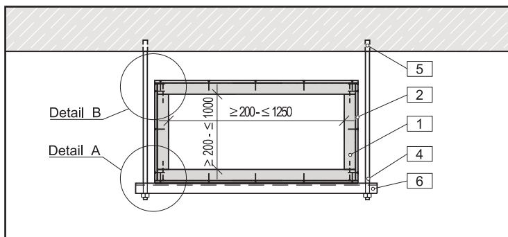
[3] Querschnitt
