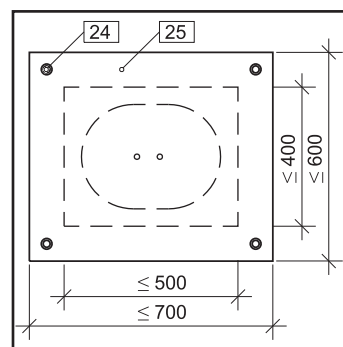
[20] Ansicht Zugangsklappe
