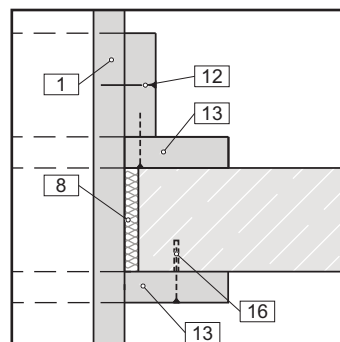
[14] Deckendurchführung, Var. 1
