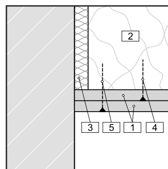
[5] Wandanschluss, Var. 2
