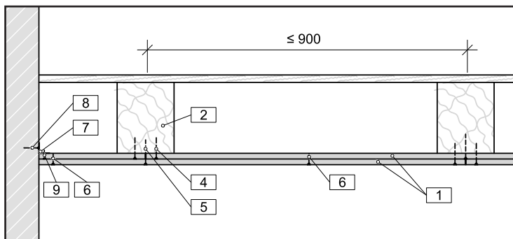
[2] Schnitt Holzbalkendecke
