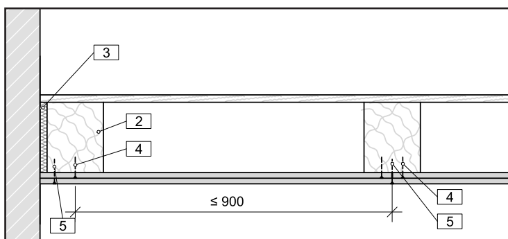
[4] Alternativer Deckenaufbau
