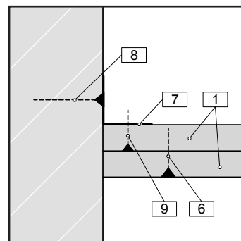
[3] Wandanschluss
