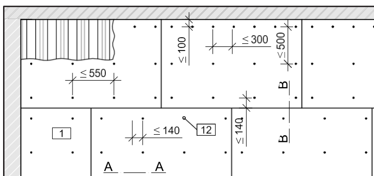
Plan du plafond réfléché
